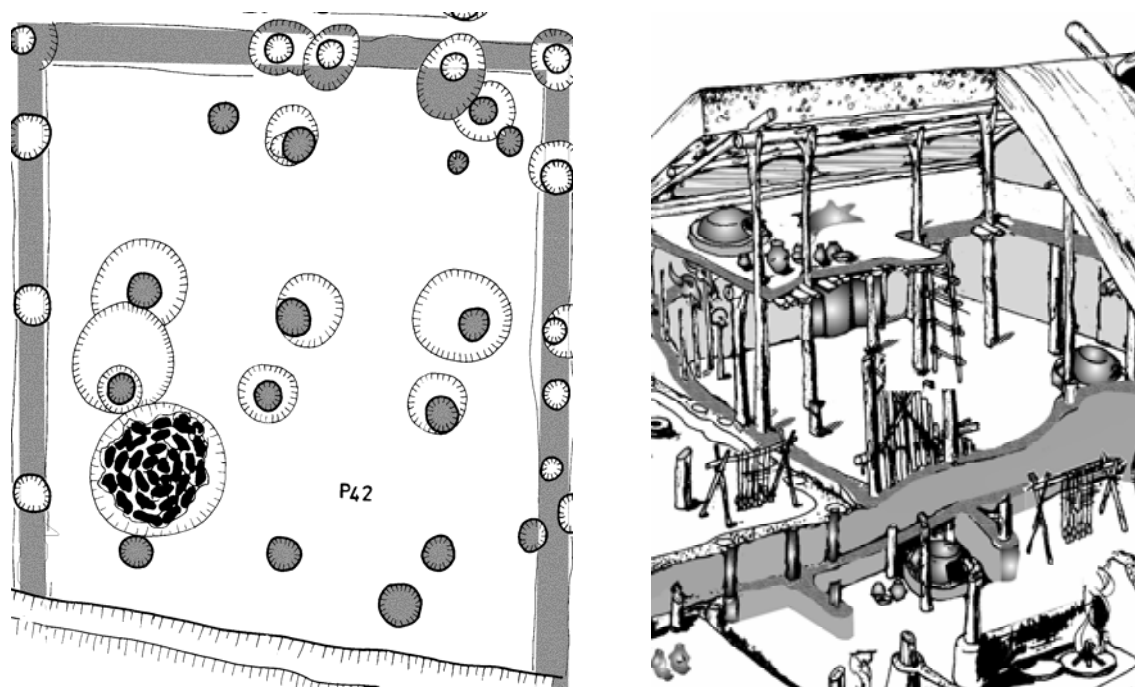
Fig. IIIb.44. Parja, Blocul Lunii, L 42: a)▲ funda]iile locuin]ei, nivel 7c; b)▲ parter [i etaj, reconstituire
