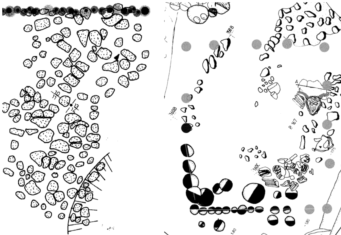
Fig. IIIb.52. Parja: a) Casa Cerbului, structura podelei, încaperea A, chirpiciul etajului; b) structură de fundație, locul capului de cerb, încaperea B
