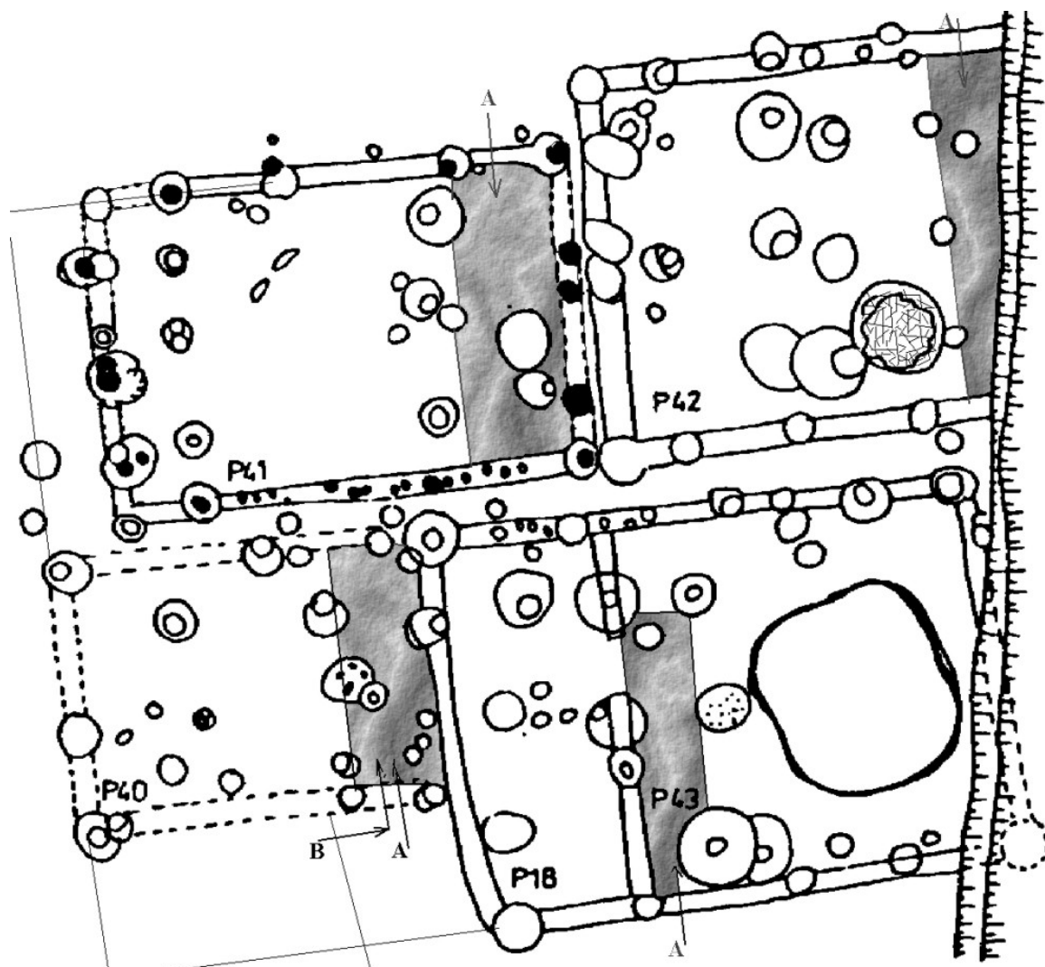
Fig. IIIb.38. Parja, bloc L40-43. Intrarea în tindele la cele patru construcții erau dinspre sud (marcate cu săgeți A și B când erau schimbări de direcție)
