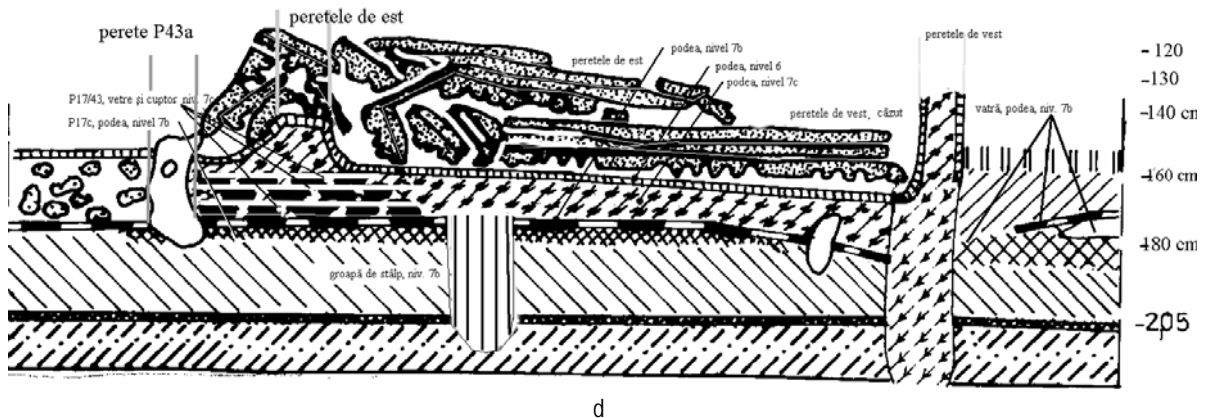
Fig. IIIb.48. Par]a, pere]ii L17: a) de vest; b) ▲ vatra central\; c) cuptorul din tind\▲; d) profil central prin vatr\▼
