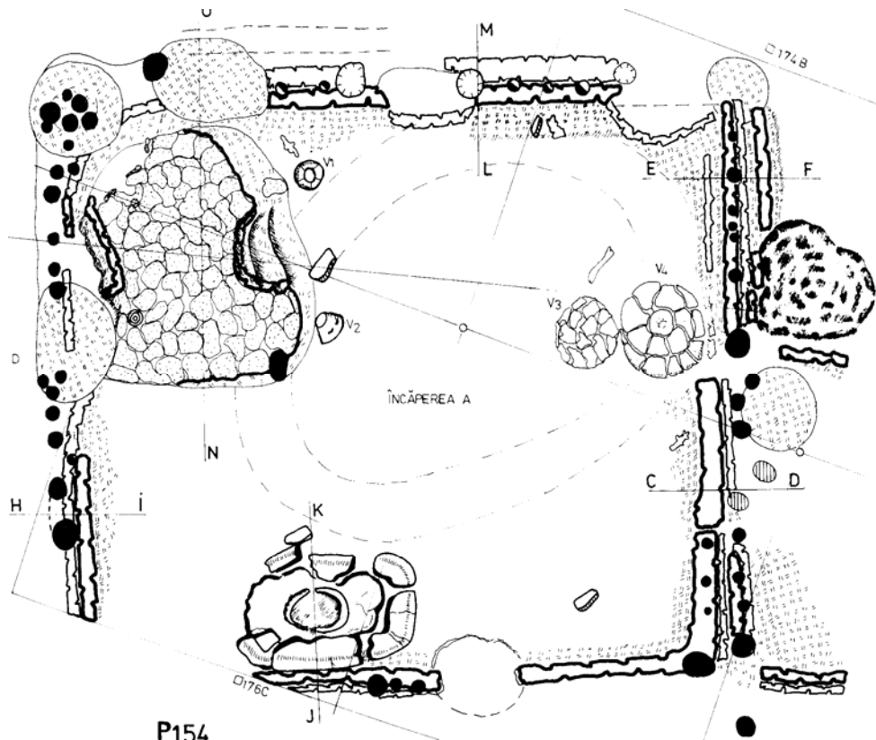
Fig. IIIb.50. Parja: a) ▲ Locuința 154; b) reconstituire ▼
